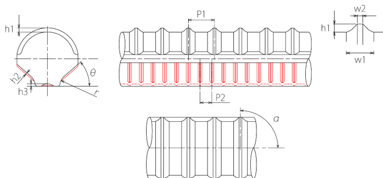
図 1 開先付き異形棒鋼の姿図
